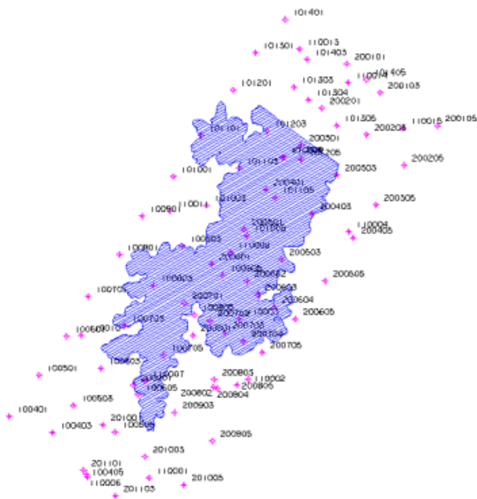
ESQUEMA DE AEROTRIANGULAÇÃO
